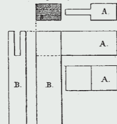
Assemblage en fourche.
